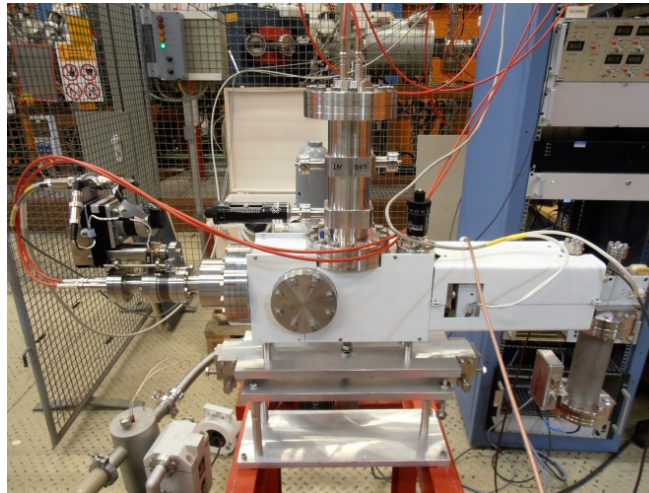
BSM CW-linac
